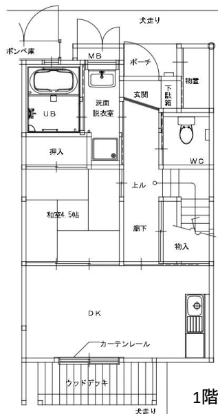
駒下アパート 2DK-B(11-105)
