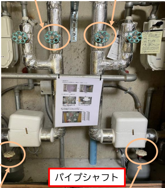
② 水抜弁 (1,3,5号室)
