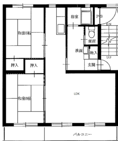
2LDK-B(13-44)
