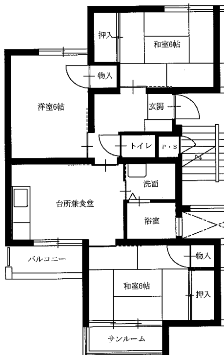
3DK(2-302)
