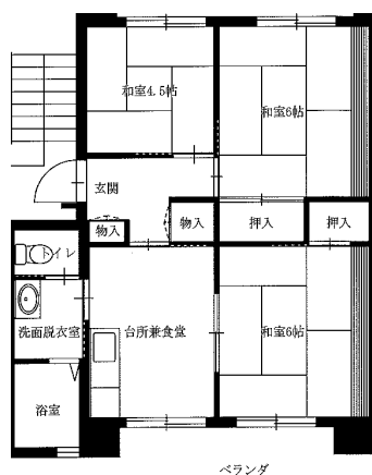
3DK(9-401) ※単身入居可
