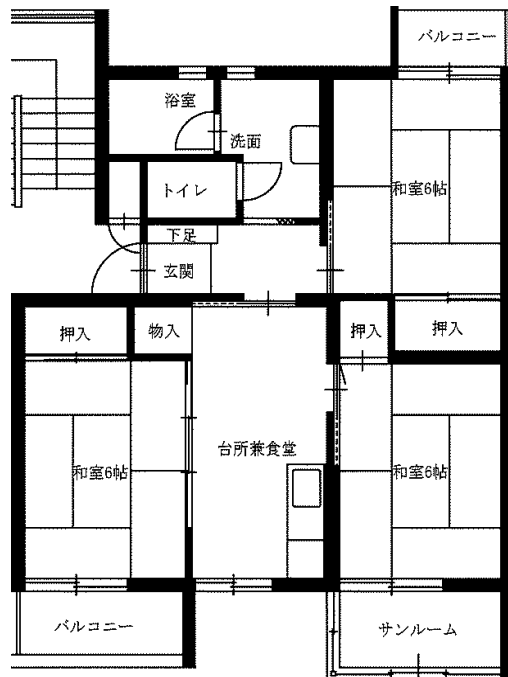
間取図
