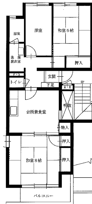
間取図
